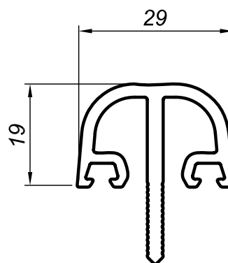
Крышка статического соединителя PC 609
