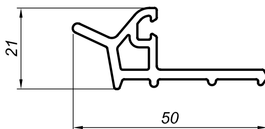
Профиль среднего уплотнения SM 50/21
