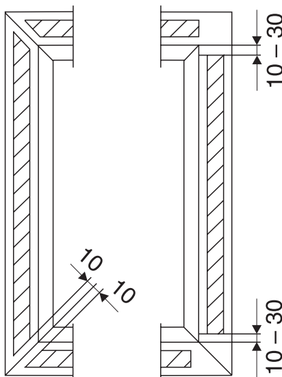
Примеры установки усиительных вкладышей
