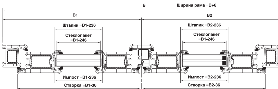
Сечение C-C
