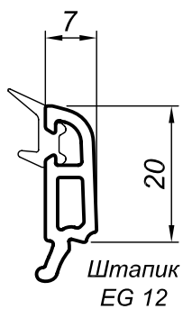
Штапик EG 12 под стеклопакет 32мм
